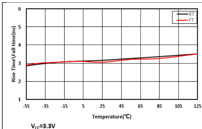
图 7-16. 驱动器输出上升/下降时间与温度
