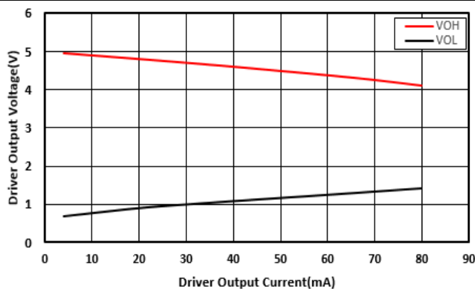
图 7-1. 驱动器输出电压与驱动器输出电流
