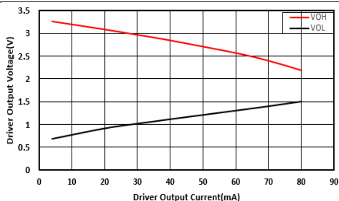
图 7-1. 驱动器输出电压与驱动器输出电流
