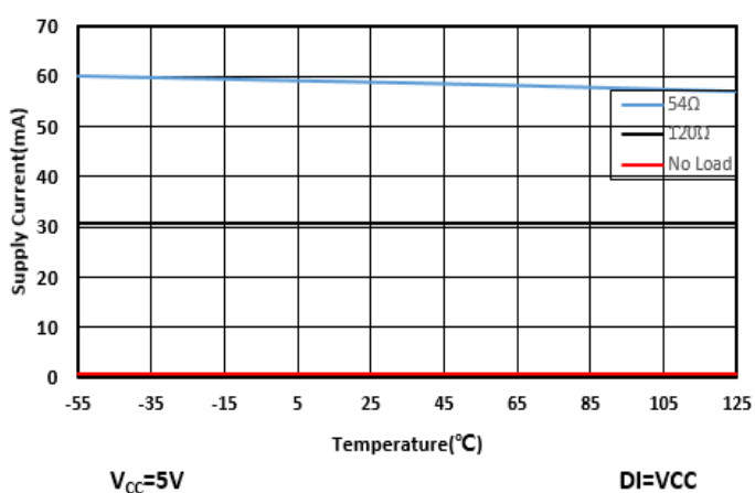
图 7-8. 静态电流与温度
