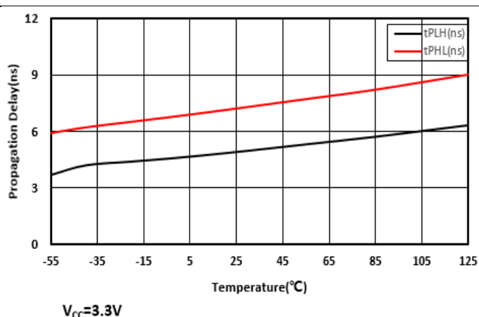
图 7-17. 驱动器传输延时与温度
