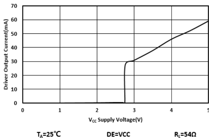
图 7-9. 驱动器输出电流与电源电压
