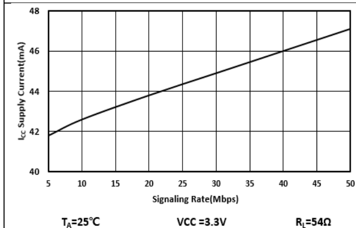
图 7-18. 电源电流与数据速率
