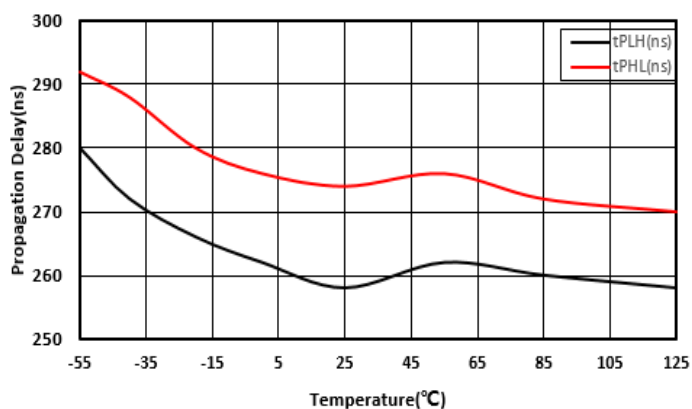
图 7-11. 驱动器传输延时与温度
