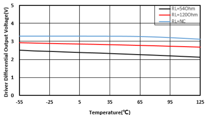
图 7-5. 驱动器差分输出电压与温度
