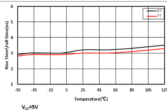
图 7-19. 驱动器输出上升/下降时间与温度
