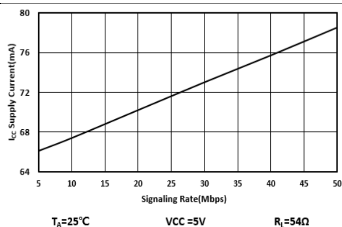
图 7-21. 电源电流与数据速率
