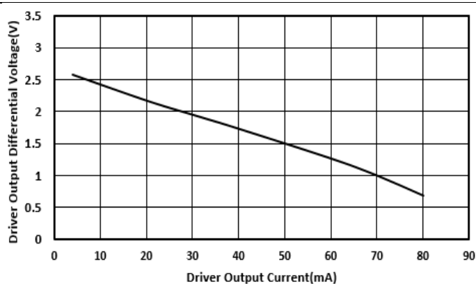
图 7-2. 驱动器差分输出电压与驱动器输出电流
