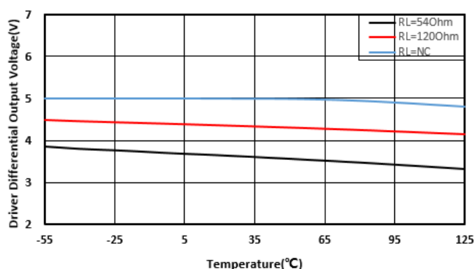
图 7-6. 驱动器差分输出电压与温度
