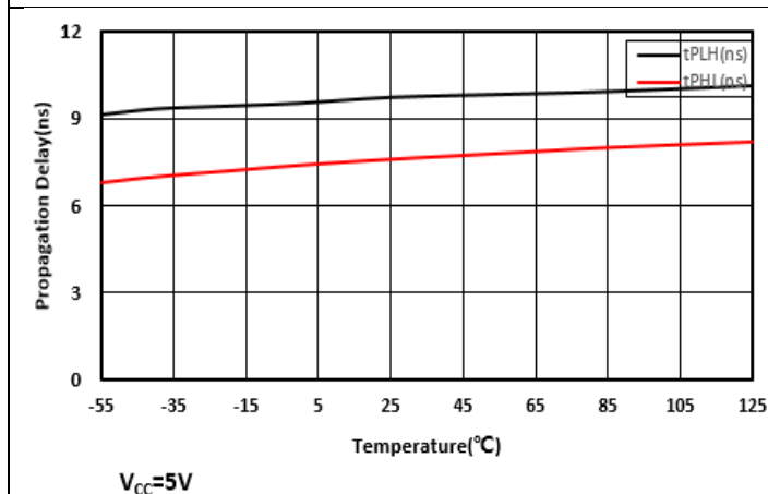
图 7-20. 驱动器传输延时与温度
