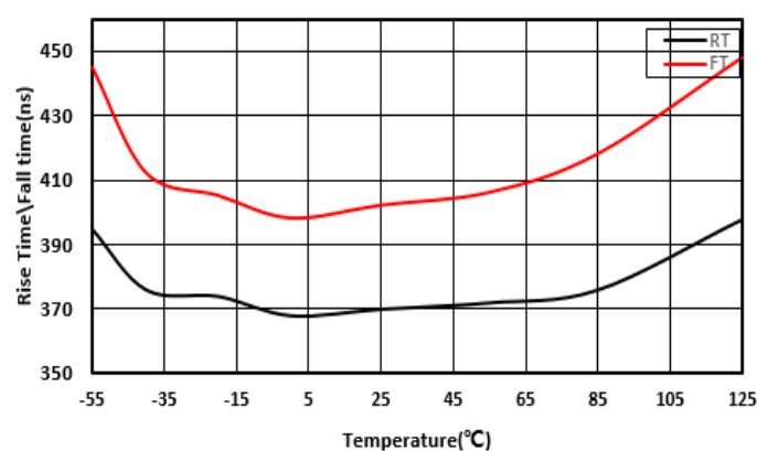
图 7-10. 驱动器输出上升/下降时间与温度
